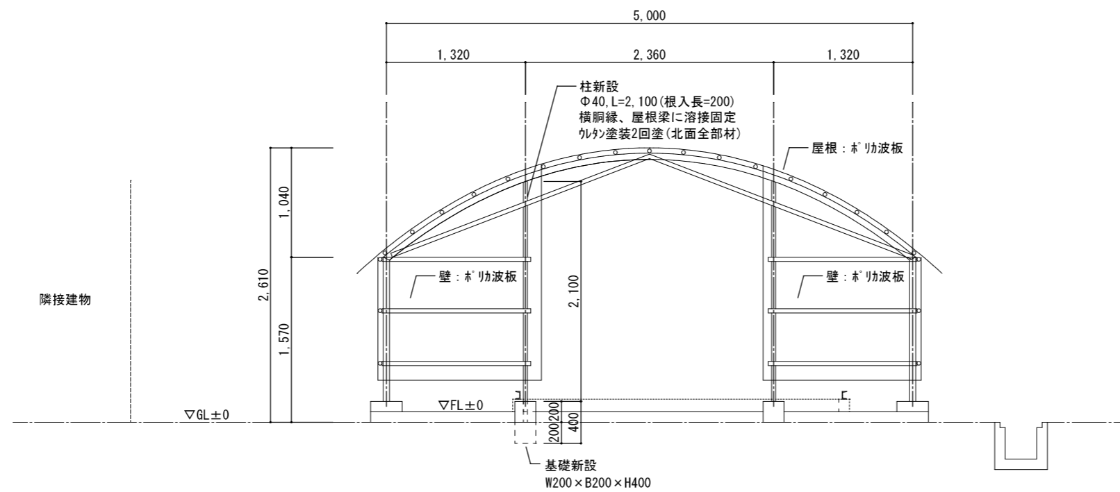
北側立面図(改修後) S=1/50
