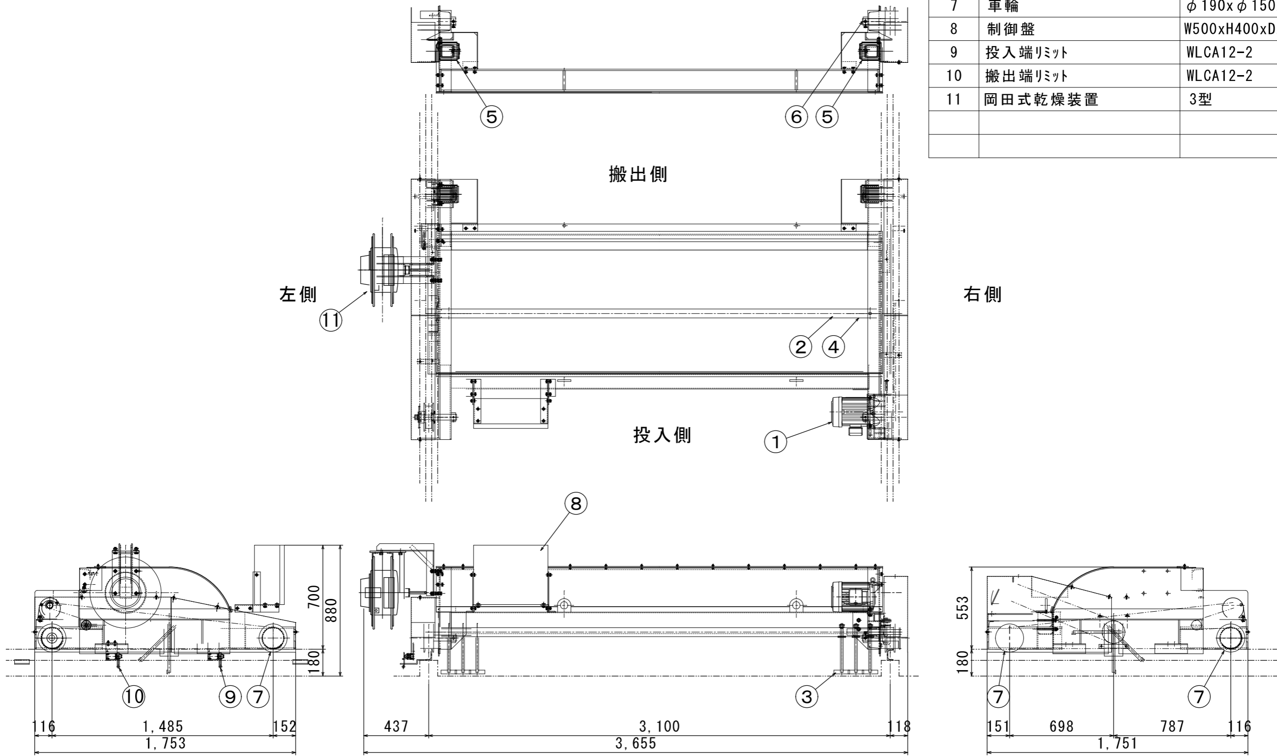
乾燥処理装置詳細図
