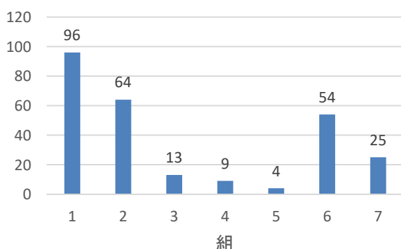
貸出冊数(1年)
