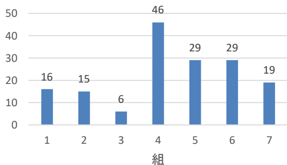
貸出冊数(3年)
