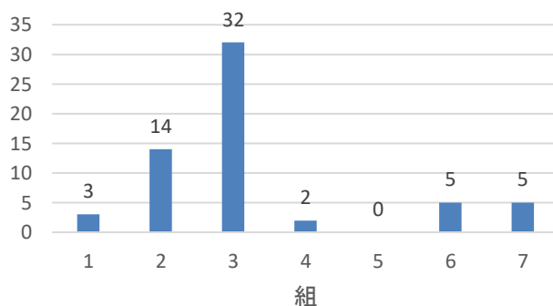
貸出冊数(2年)
