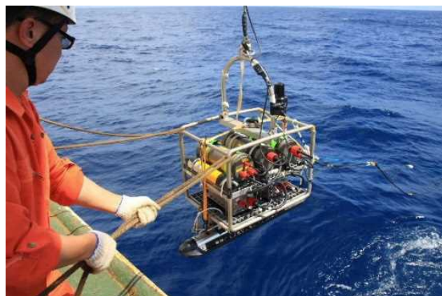
図 2. 海底電気探査の模式図（左）と実機（右）。深海曳航に電流送信装置を搭載し、その後方に電流送信・電圧受信用電極を多数曳航しながら、海底下の比抵抗構造を連続的にスキャンできる。
