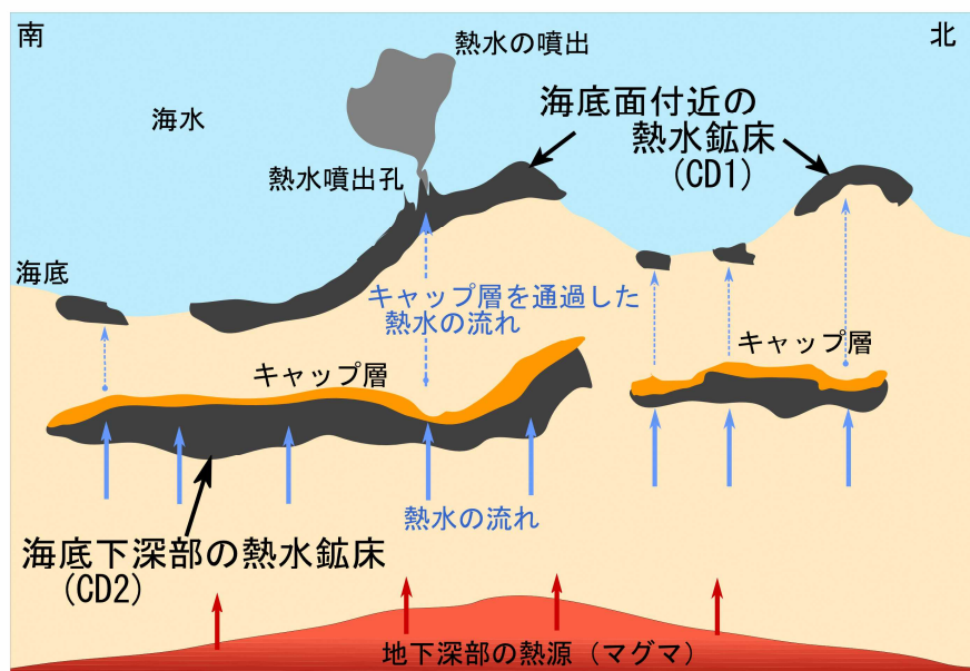
図：本研究で提案された「二階建て」の熱水鉱床の形成メカニズム
