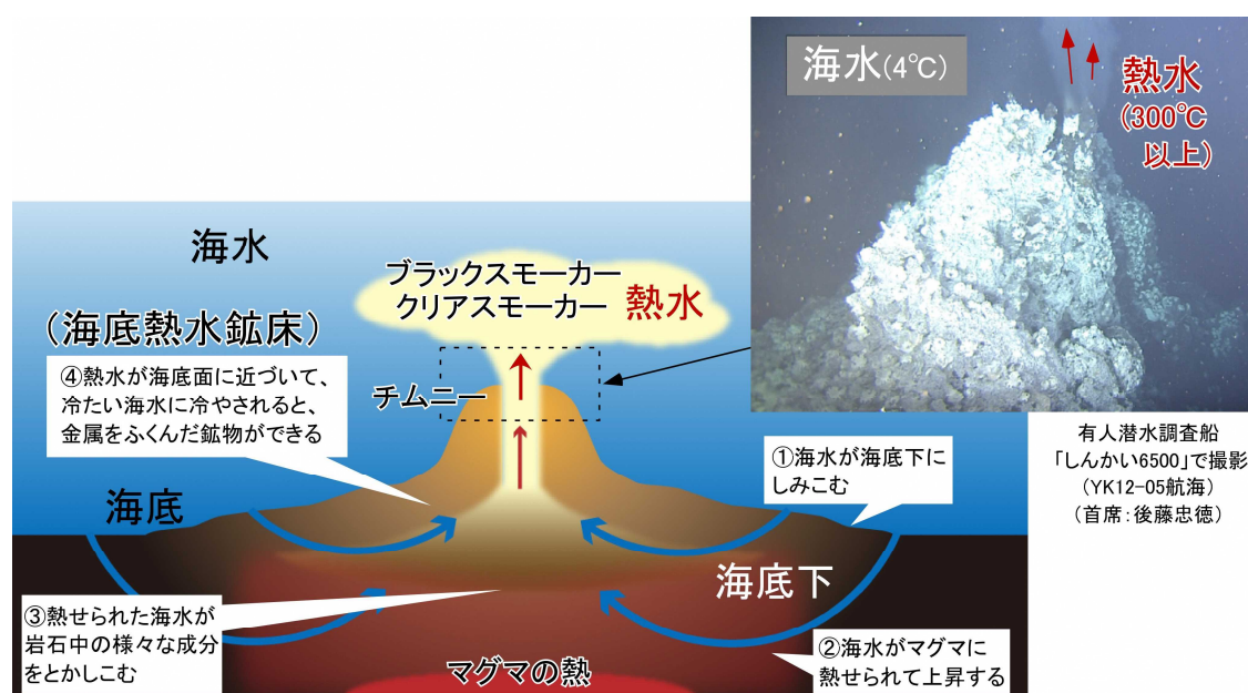
図 1. 海底熱水鉱床の形成メカニズムの模式図（写真は海底熱水噴出孔）右記ページの図に加筆 ( www.jamstec.go.jp/j/kids/press_release/20120323/ )。ただし、具体的なメカニズムは不明だった。
