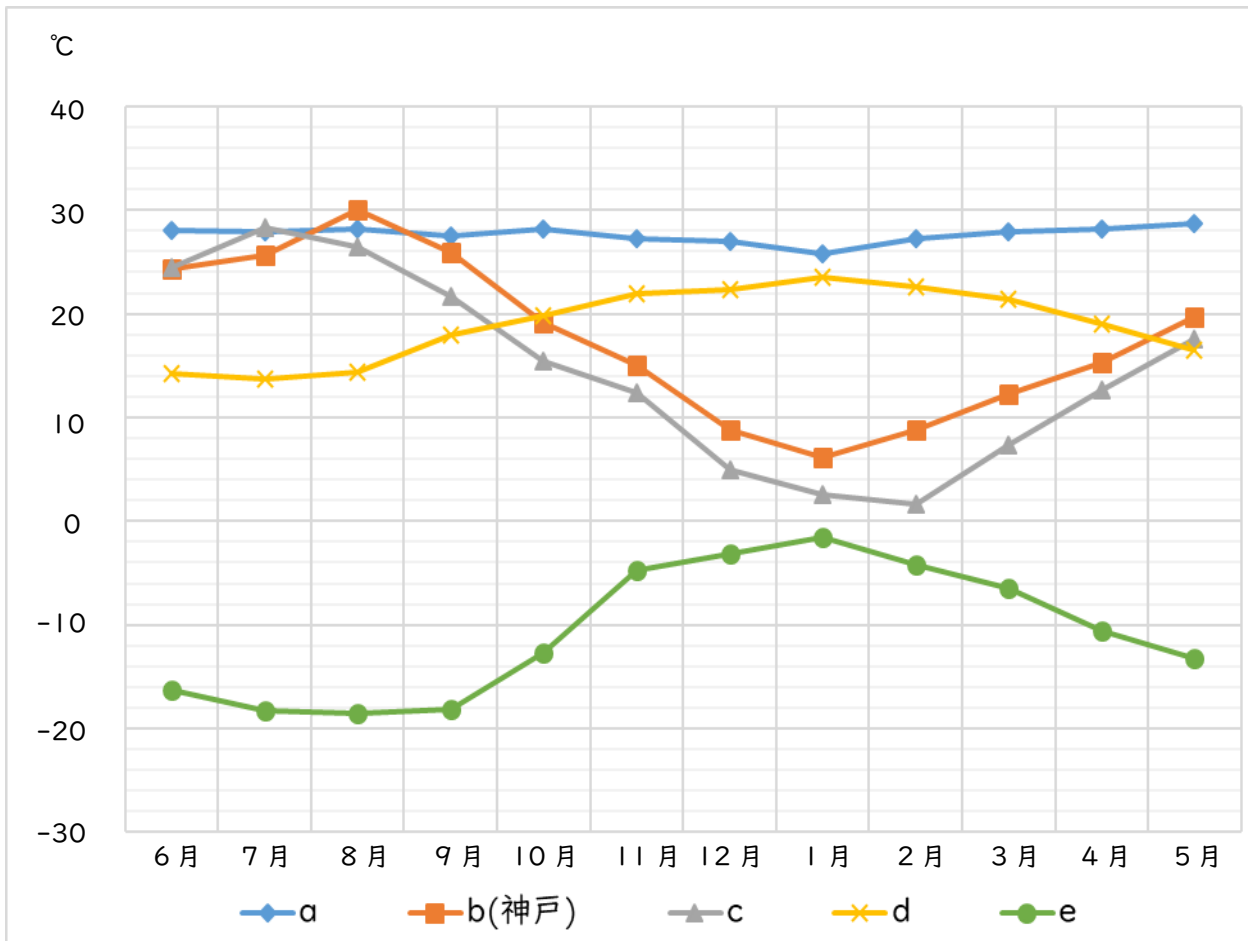
【資料3 各地点別月平均気温グラフ】
