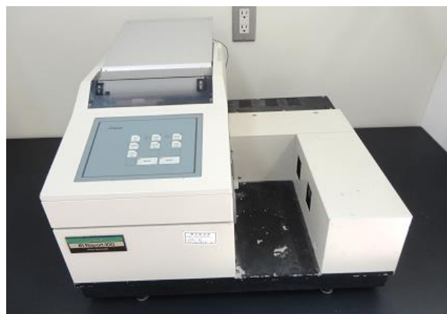
赤外分光光度計 Jasco IR Report-100
